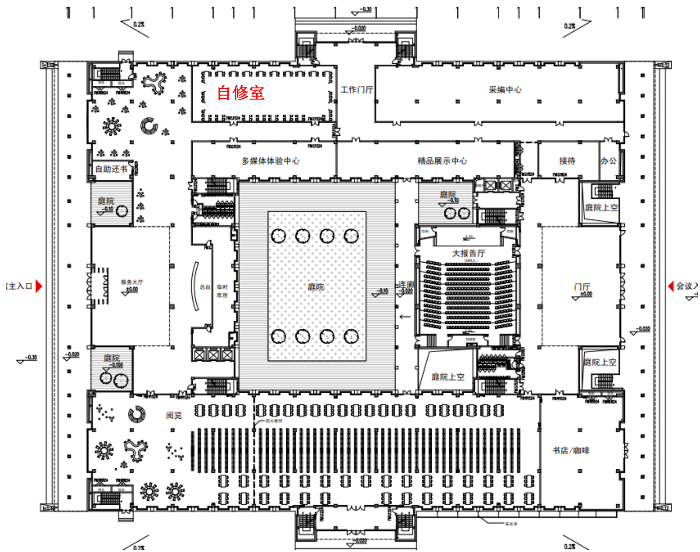
▲ 一楼平面图
