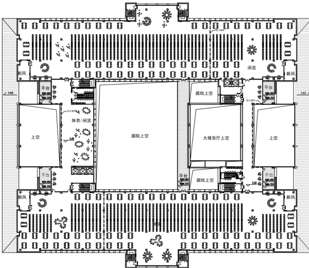
▲ 二楼平面图
