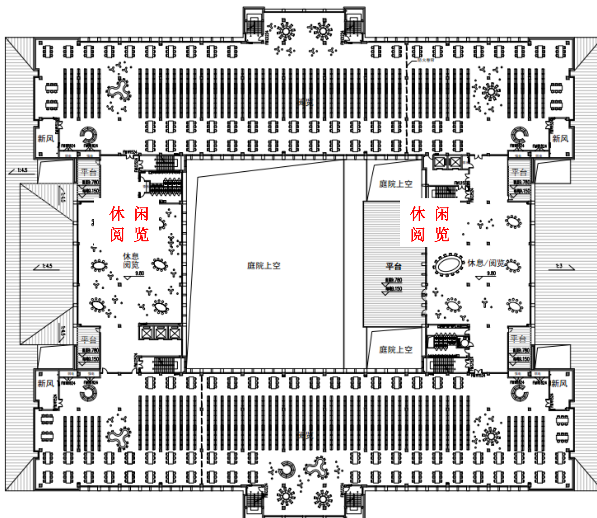
▲ 二楼平面图
